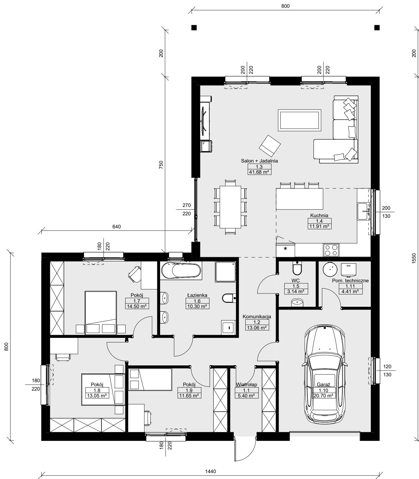
RZUT PARTERU 1 : 100
